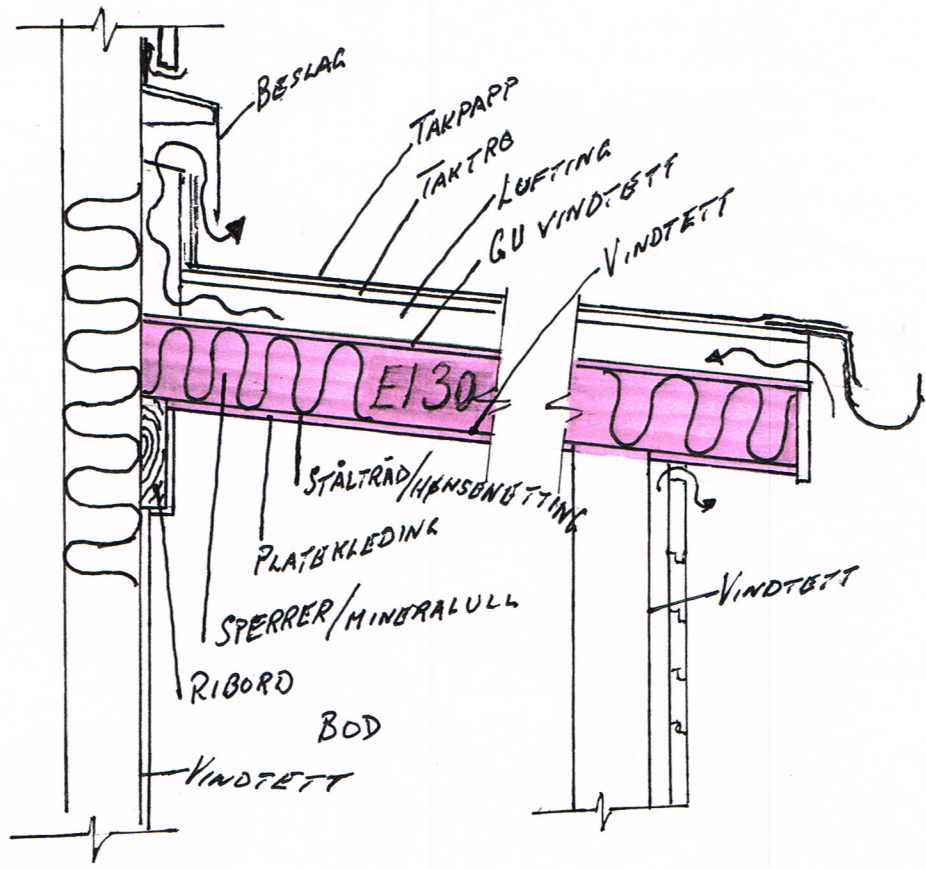
SNITT EKSEMPEL TAK/VEGG
